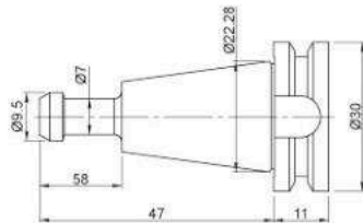
BT20 刀桿錐度尺寸 BT20 SHANK INFORMATION
