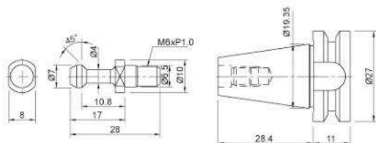
BT15 刀桿錐度尺寸 BT15 SHANK INFORMATION
